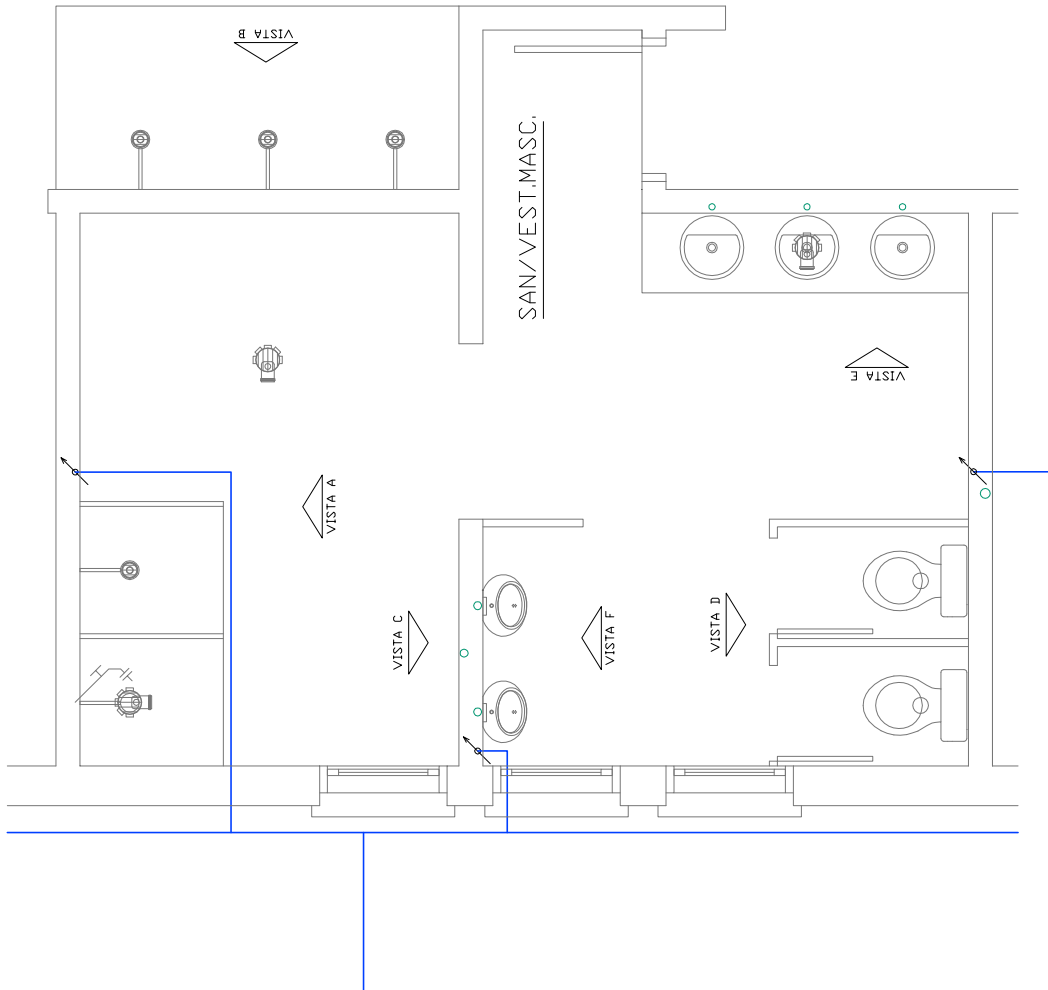
PLANTA BAIXA
