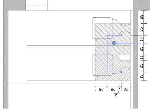
VISTA B
