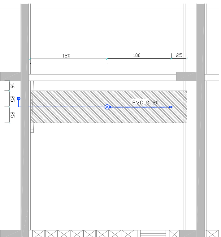
PLANTA BAIXA
