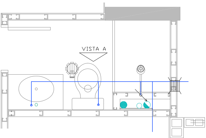
PLANTA BAIXA
