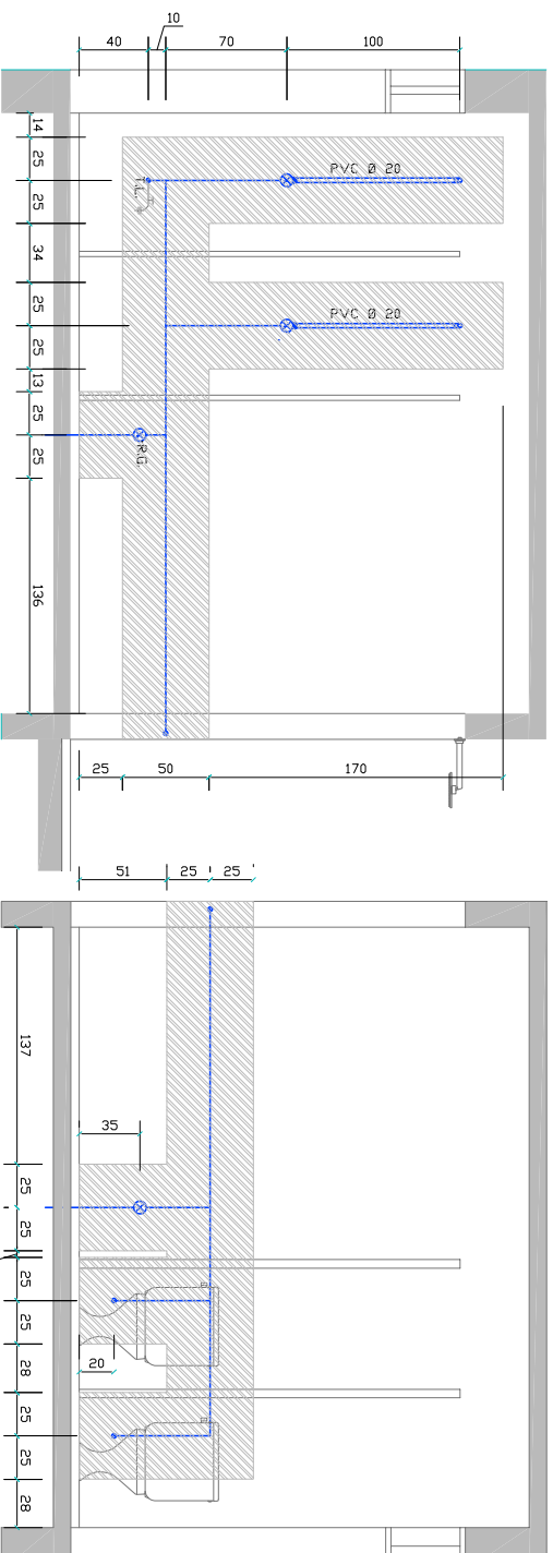
VISTA D
