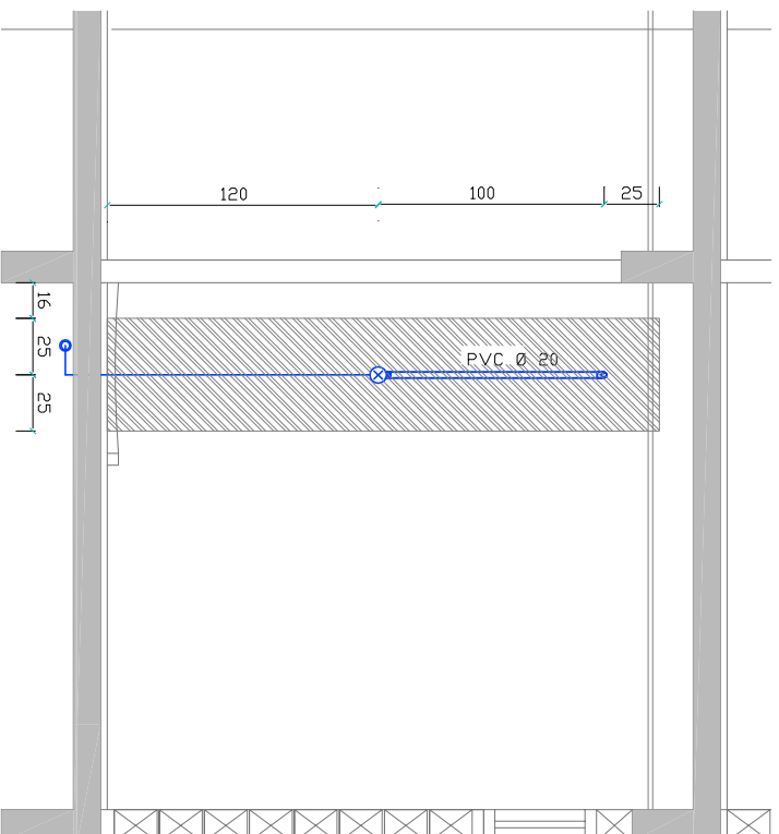
PLANTA BAIXA
