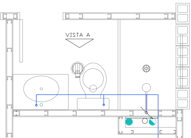
PLANTA BAIXA
