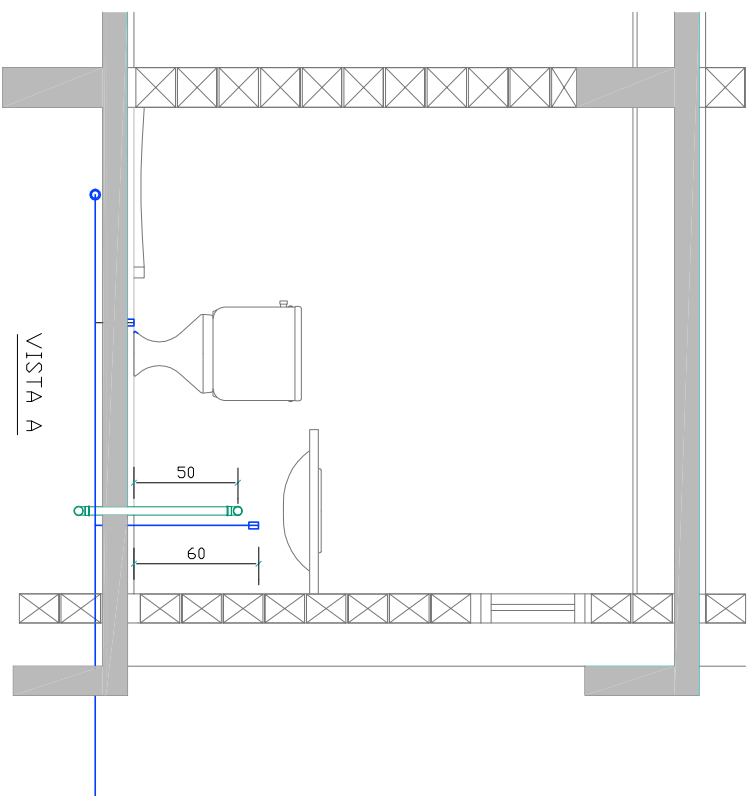
PLANTA BAIXA
